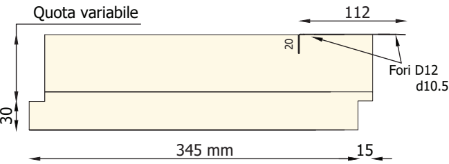
vista alto
