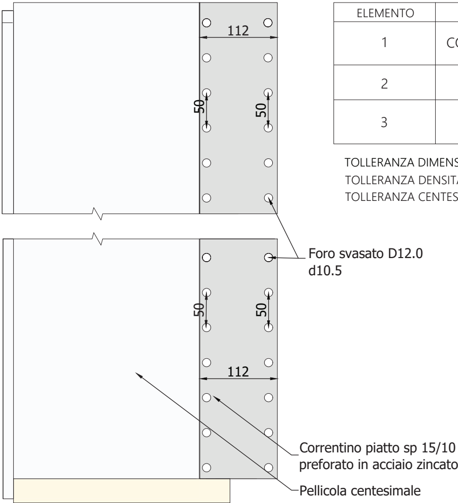
vista alto
