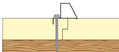
Fissaggio del pannello FibroTek
