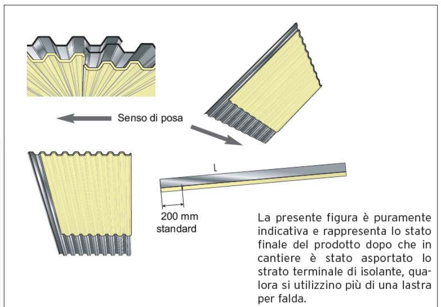
sovrapposizione laterale di una greca e mezzo
