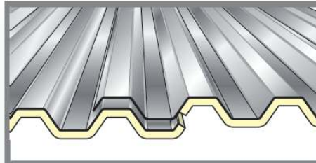
sovrapposizione laterale di una greca e mezzo
